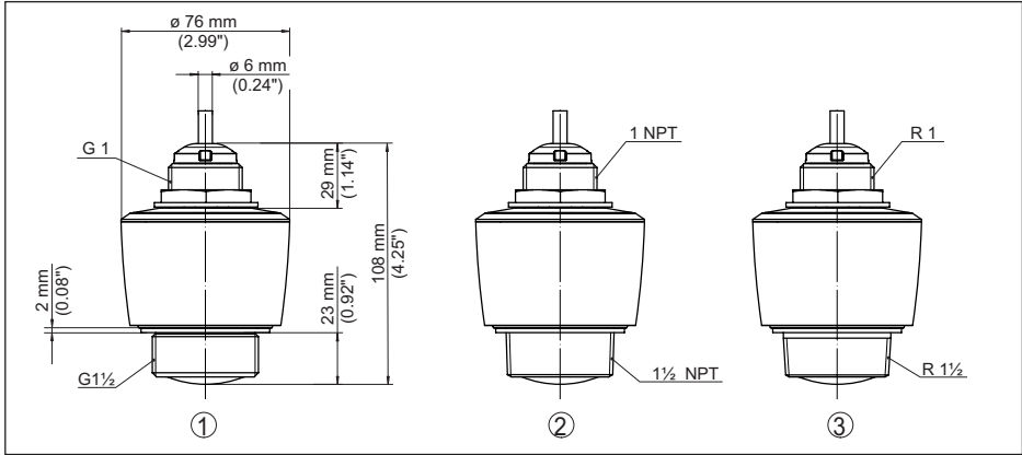
도면. 27: 크기 VEGAPULS C 11
