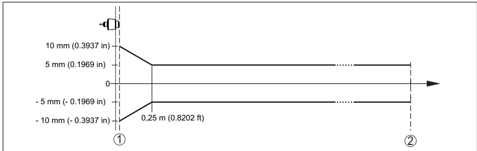
도면 26: 기준 조건에서 측정 편차 7)
