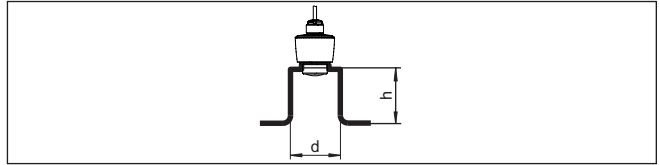
도면. 10: 파이프 노즐 치수가 다른 경우 파이프 노즐 장착
