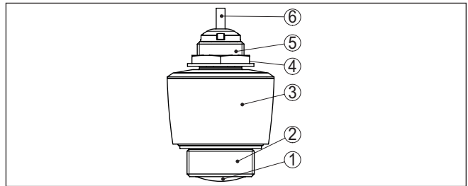
도면 1: VEGAPULS C 11의 구성요소
