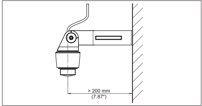
도면 3: 설치 브래킷을 통한 장착
