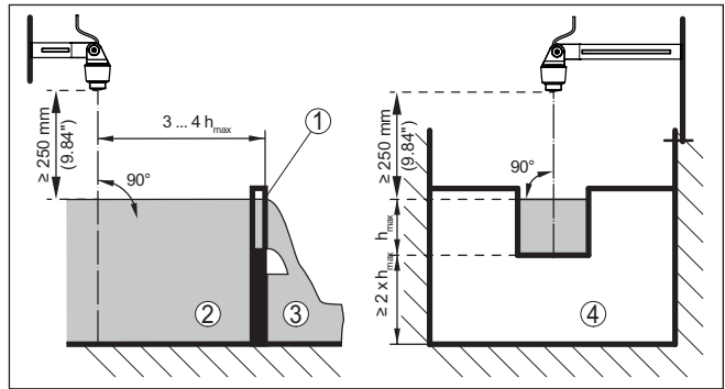
도면. 16: 직사각 플룸의 유량 측정: h_{\max} = 직사각 플룸의 최대 총입량
