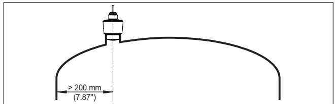
도면 5: 둥근 용기 천장에 레이더 센서 장착하기
