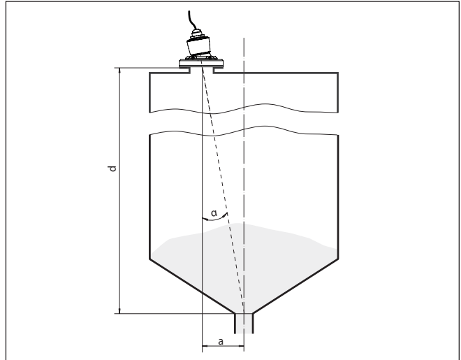
도면. 14: VEGAPULS C 11 정렬 후 설치 제안
