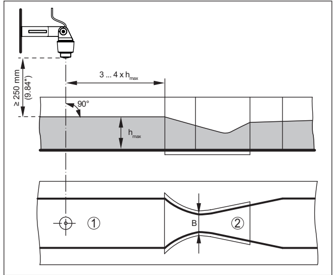
도면. 17: Khafagi-Venturi 플룸을 사용한 유량 측정: h_{\text{max}} = 플룸의 최대 총입량; B = 플룸의 최대 협착량
