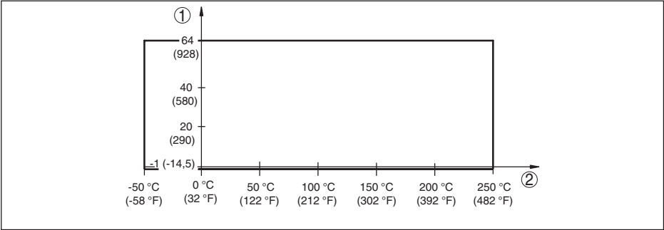
도면. 17: 공정 온도 - 스위치 위치 \geq 0.7 \text{ g/cm}^3 경우 공정 압력(감도 스위치)
