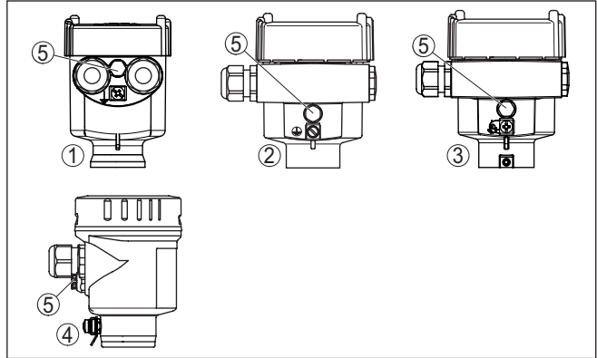
도면. 9: 싱글 챔버 하우징 재료 버전
