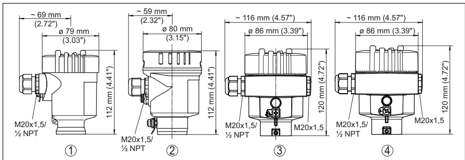
도면: 19: 하우징 버전
