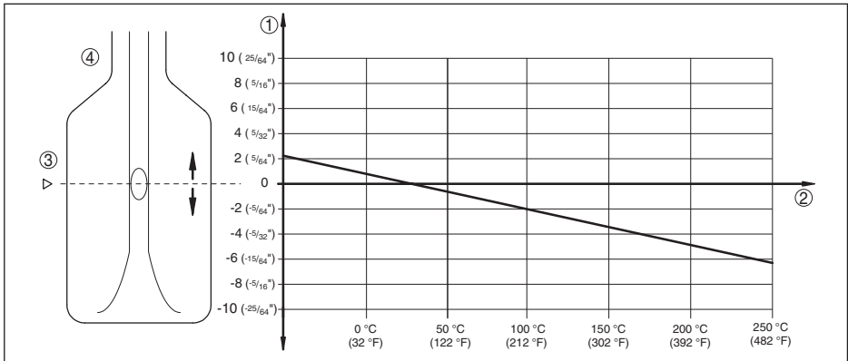
도면. 13: 스위칭 포인트에 공정온도의 영향
