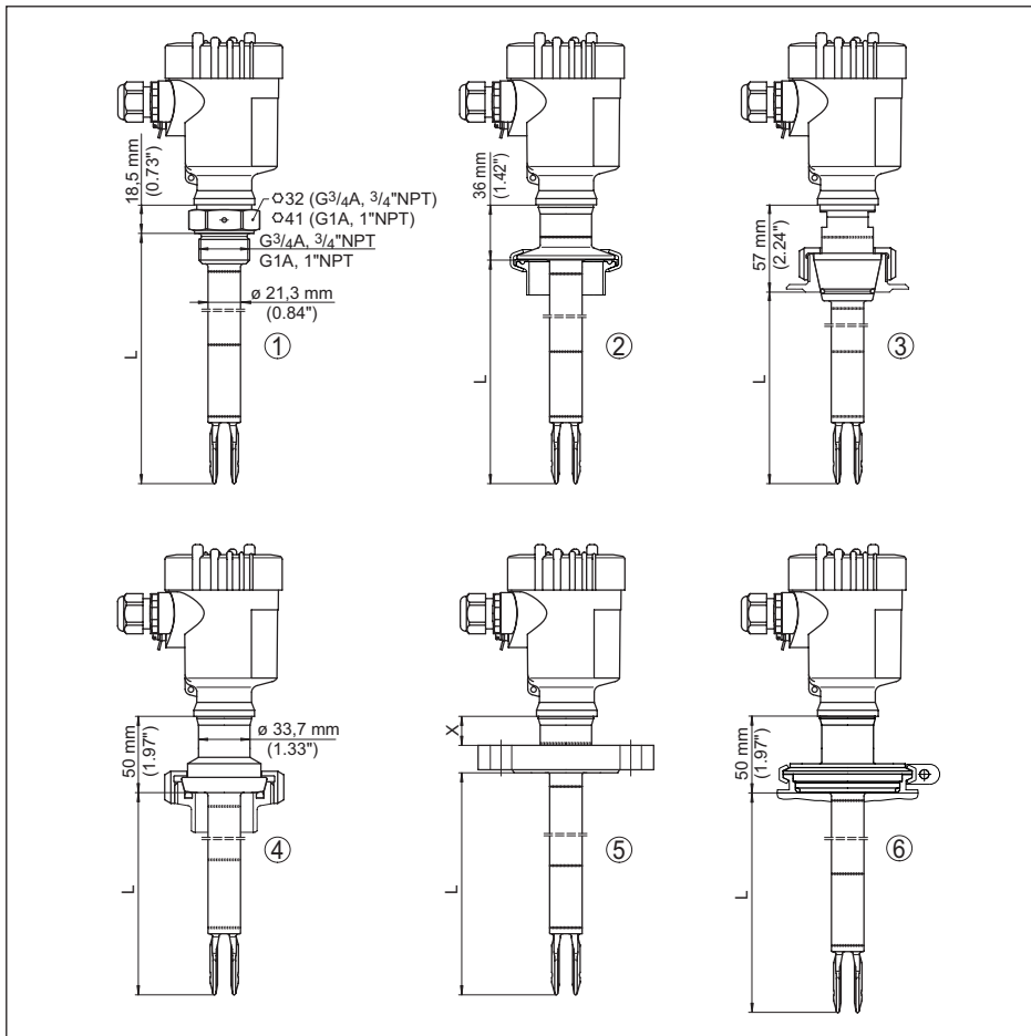
도면. 20: VEGASWING 63
