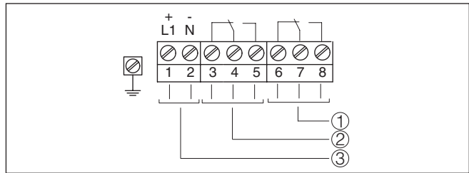
도면. 11: 결선도, 상글 챔버 하우징
