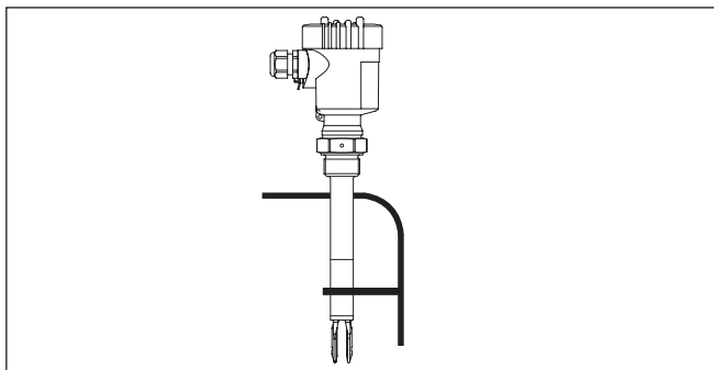
도면 8: VEGASWING 63의 측면 지지대
