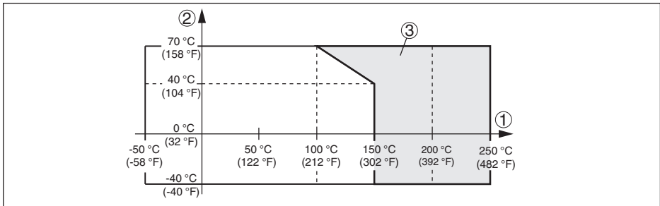
도면. 16: 주변 온도 - 공정 온도
