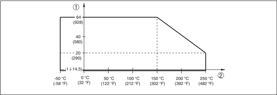
도면. 18: 공정 온도 - 스위치 위치 \geq 0.5 \text{ g/cm}^3 경우 공정 압력(감도 스위치)
