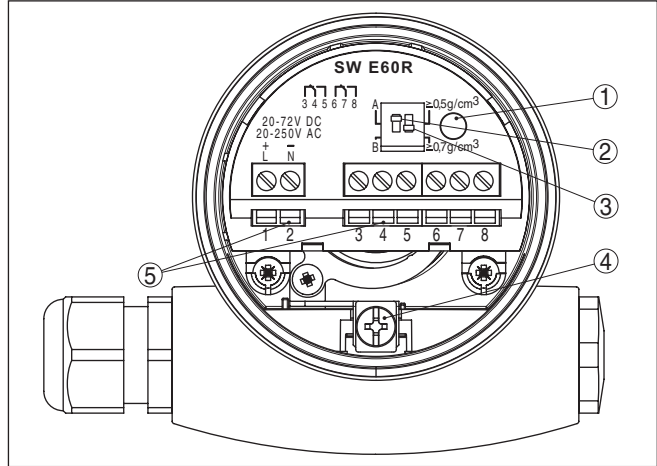
도면. 10: 전자장치 및 연결장치 공간 상글 챔버 하우징
