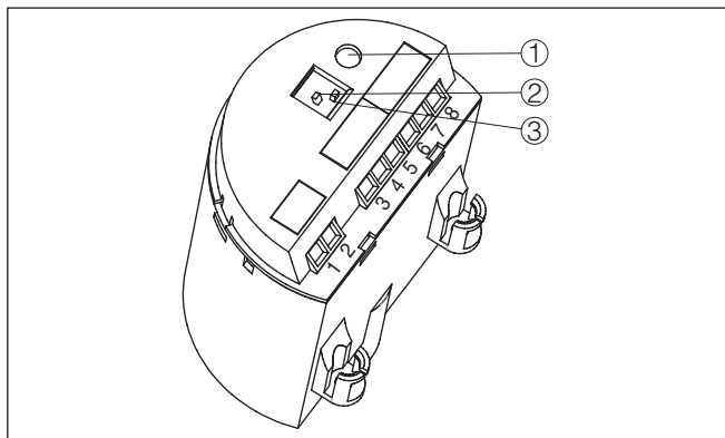
도면. 12: 일렉트로닉 모듈 SWE60R - 릴레이 출력
