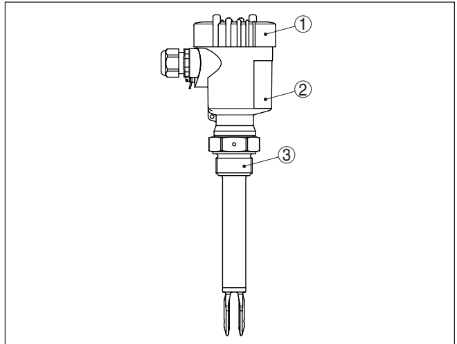
도면. 1: VEGASWING 63
