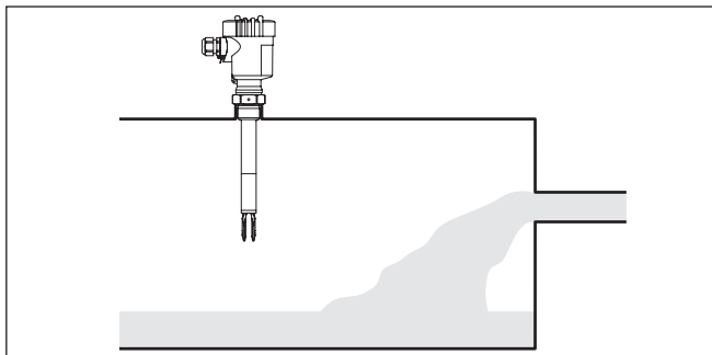
도면 7: 유입하는 매질
