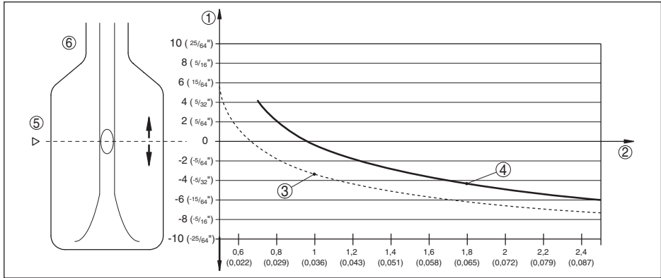
도면 14: 스위칭 포인트에 충입물 밀도의 영향
