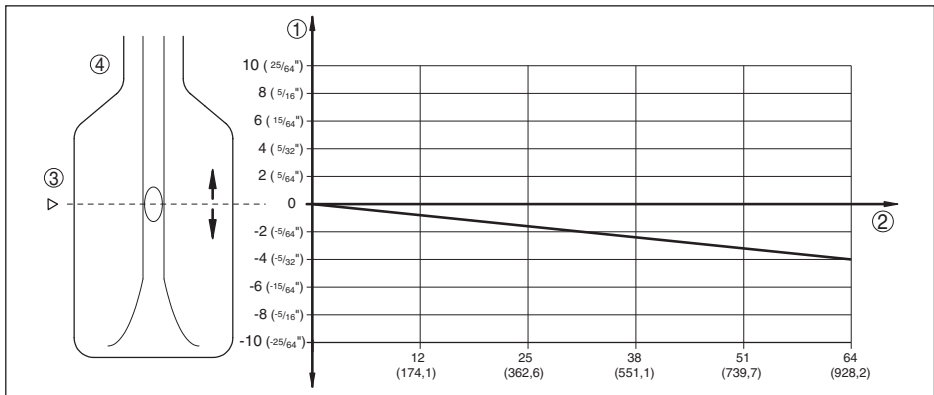
도면 15: 스위칭 포인트에 공정압력의 영향
