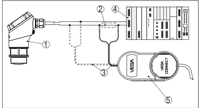
도면. 29: PC를 신호 케이블에 연결
