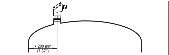
도면. 6: 둥근 용기 천장에 레이더 센서 장착하기
