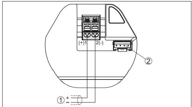
도면. 19: 연결구획 VEGAPULS 31
