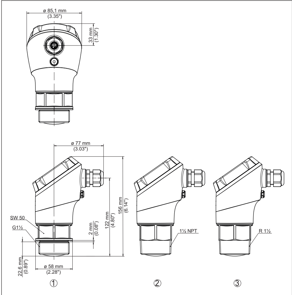
도면. 36: 크기 VEGAPULS 31
