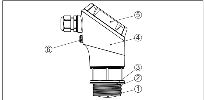
도면. 1: VEGAPULS 31의 구성요소
