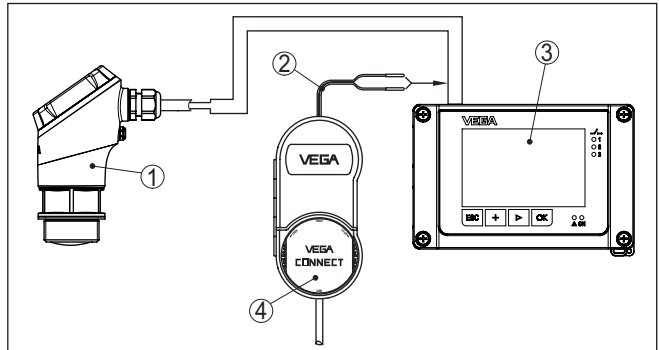
도면. 30: PC를 VEGAMET 컨트롤러에 연결하기
