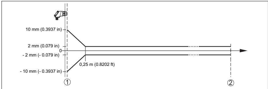
도면. 35: 기준 조건에서 측정 편차 10)
