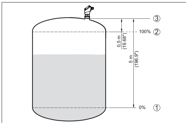
도면. 24: 매개변수 조정 예, 최소/최대 조정
