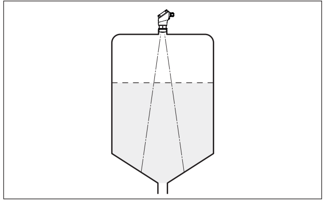
도면. 7: 원추형 바닥이 있는 용기에 레이더 센서 장착하기
