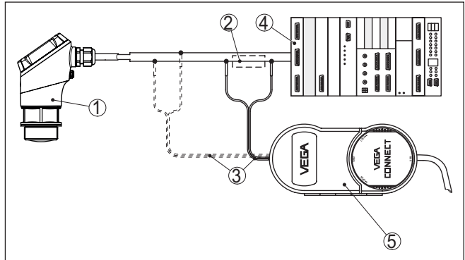
도면. 3: PC를 신호 케이블에 연결
