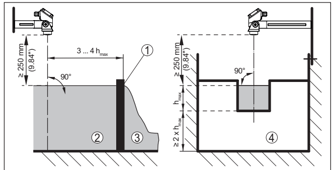
도면. 16: 직사각 플룸의 유량 측정: h_{\text{max}} = 직사각 플룸의 최대 총입량
