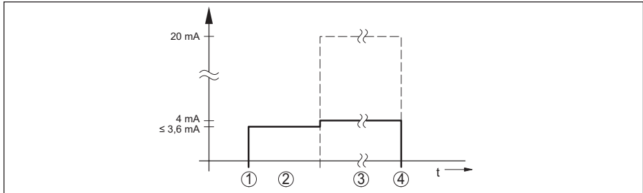
도면. 34: 가동 시간 및 측정값 출력
