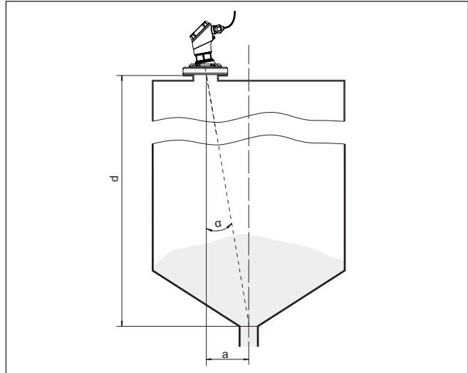
도면. 14: VEGAPULS 31 정렬 후 설치 제안
